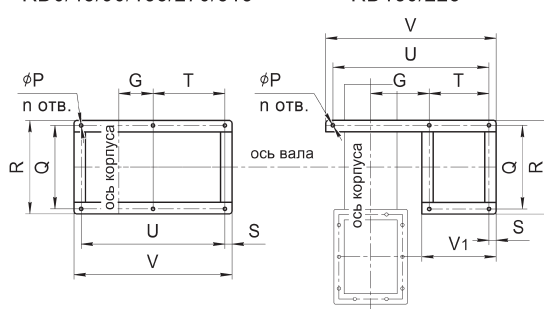
Опорная рама
