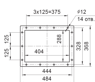
Выходной фланец
