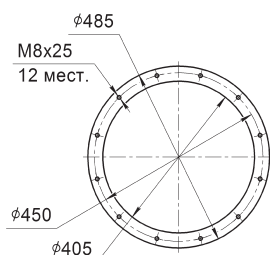
Входной фланец
