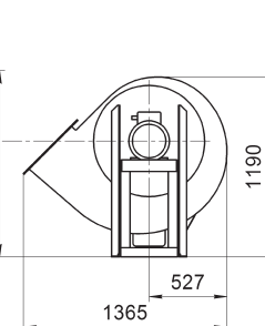
Выходной фланец
