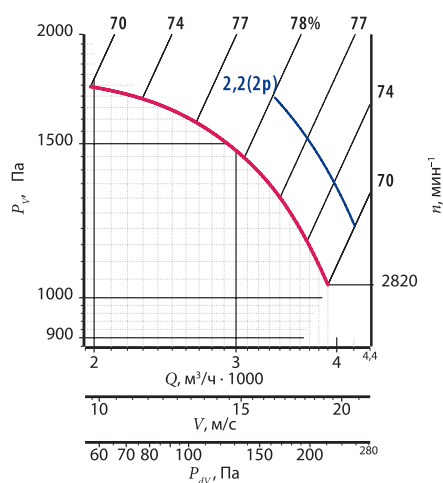
Тип вентилятора ВИР(1)-F
