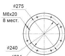
Входной фланец
