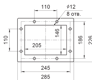
Выходной фланец
